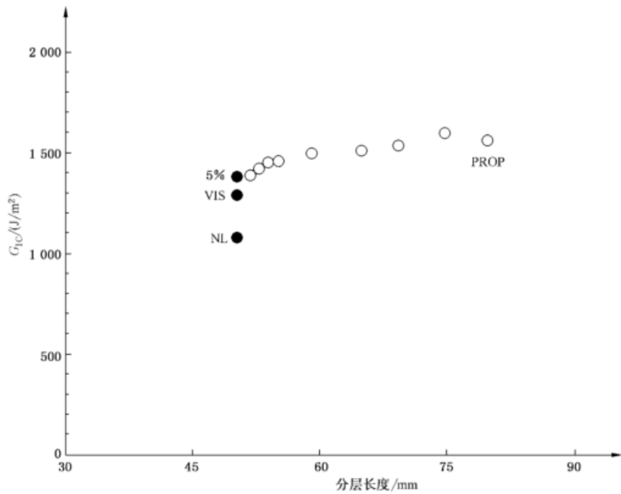
图 7 典型的分层-阻力曲线(R-曲线),分层阻抗随分层长度增加而增加
