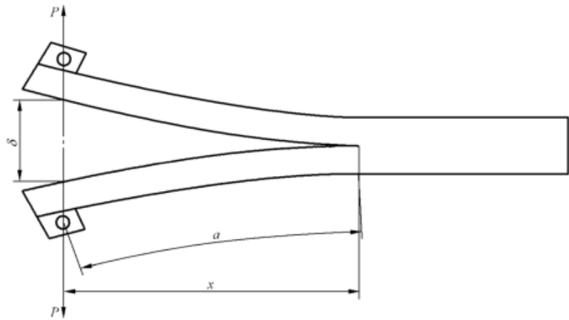
图 6 DCB 试样在加载时,沿水平方向上测量的分层长度 x ,沿固定在试样上的刻度尺方向测量的分层长度 a
